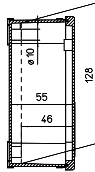
Sez. B-B
