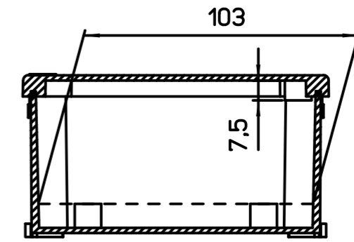
Sez. A-A
